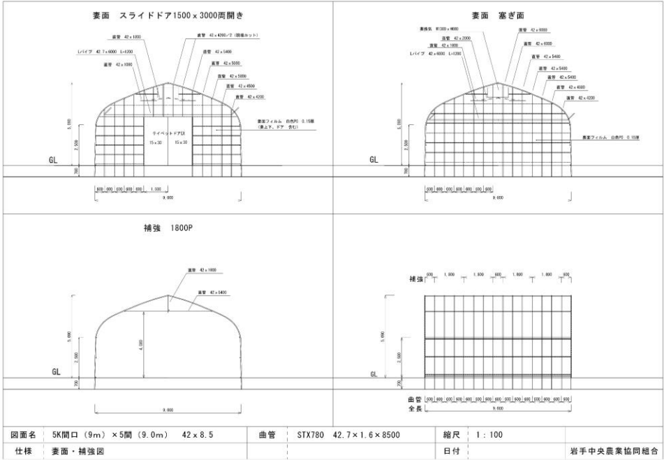
5間×5間格納庫ハウス 完成イメージ
